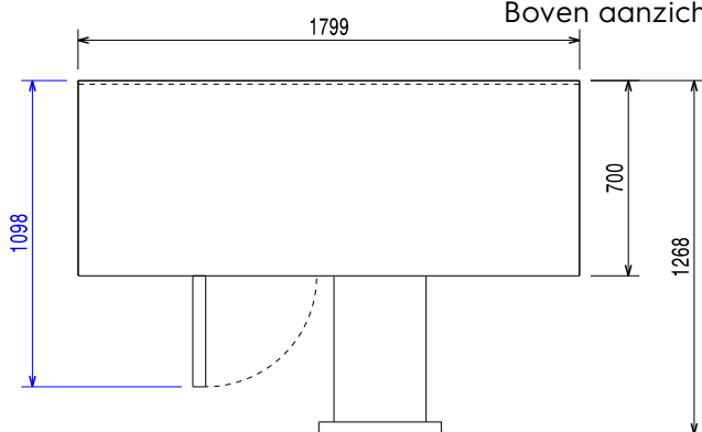
Boven aanzicht
